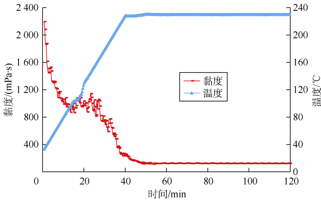
图3 230 °C超高温压裂液体体系流变特性曲线
